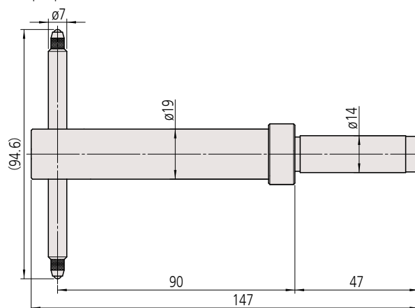
1) 12AAC072 Depth probe
